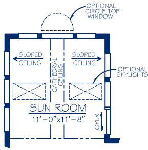
OPTIONAL SUN ROOM
